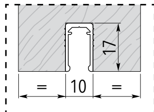
Eingesetztes Türführungsprofil
