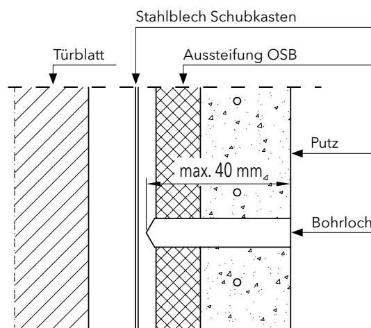
Schematischer Aufbau (Schnitt) der Seitenwand des Schiebetürkastens Mod. ECLISSE EWOLUTO®
